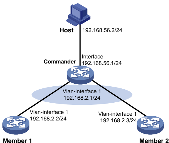
图12-6 配置 SmartMC 网络的出接口组网图
