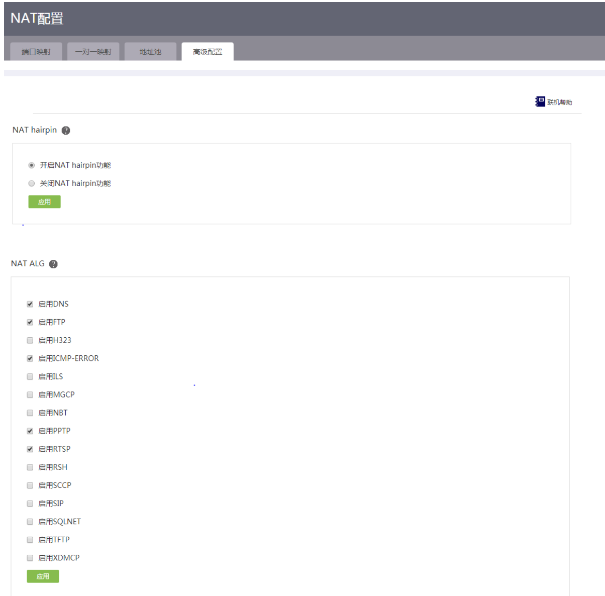
图5-19 高级配置-NAT ALG
